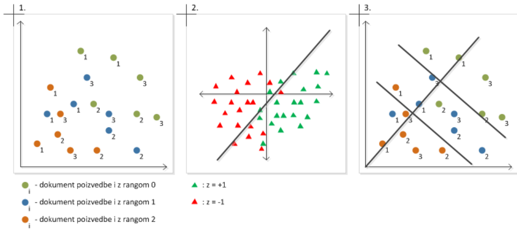
Slika 3.9: Ranking SVM primer. 1. podatki za tri poizvedbe predstavljeni v ravnini, 2. pretvorba podatkov in izračun ločitvene premice, 3. ločitvena premica med prvotnimi podatki z mejami
