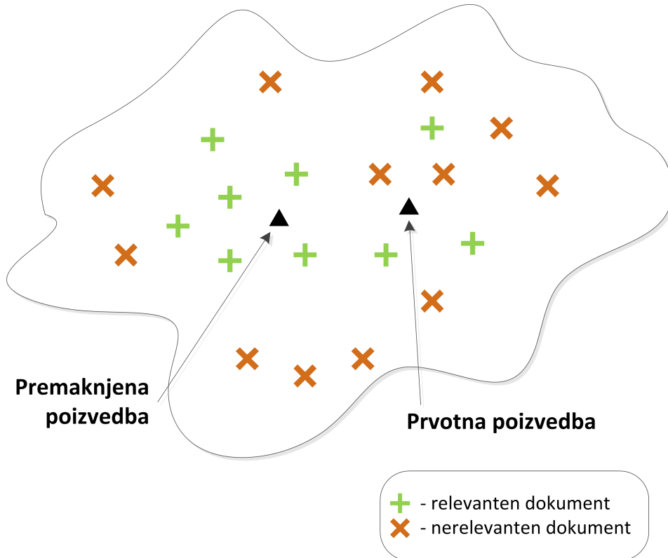
Slika 3.4: Rocchio algoritem. Algoritem predlaga bolj primeren vektor glede označene dokumente.
